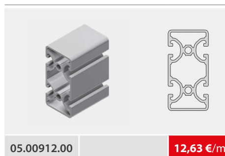
Aluprofil 40 x 80EL-2N180
