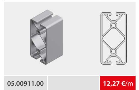
Aluprofil 40 x 80EL-4N180
