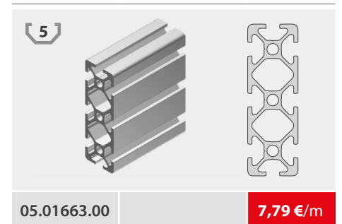
Aluprofil 20 x 60/Nut 5
