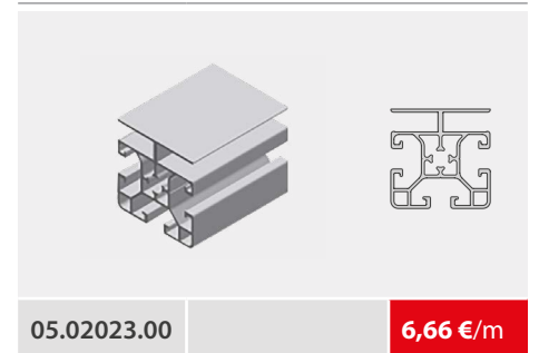
Schutzzaunprofil 40 x 40-180°
