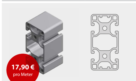
Aluprofil 40 x 80N-2N180
