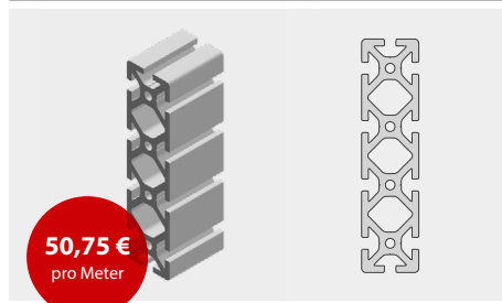
Aluprofil 40 x 160 S
