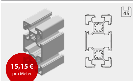
Aluprofil 45x90L-2,9
