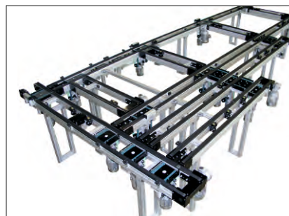
DG-2 Anlage
