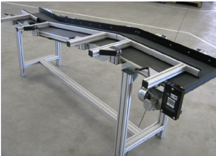
Bandförderer BF-40
