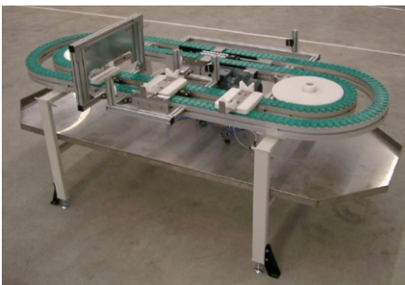
Doppel-Kunststoffkettenförderer
